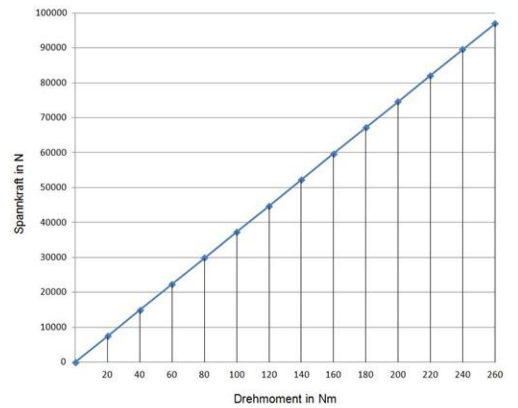
Spannkraft - Drehmoment BSMG-400
