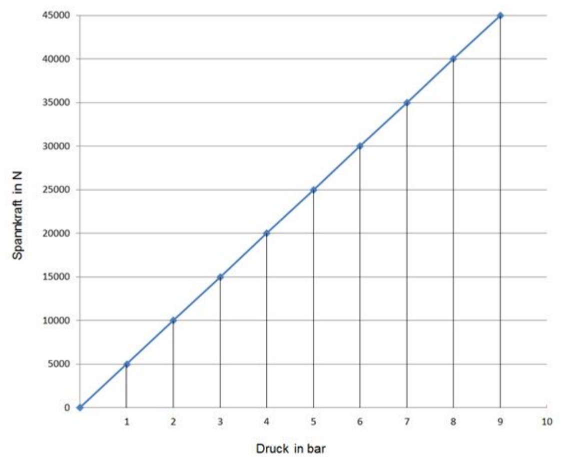
Spannkraftdiagramm BSP250
